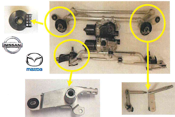
リンクユニット (ワイパー駆動部部品) ブラケットユニット (ワイパー基幹部品)
